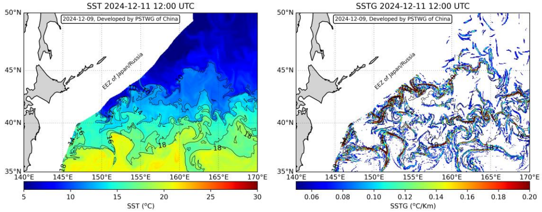
2024 年 12 月 11 日, 秋刀鱼渔场海水温度和锋面预报图
